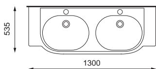
dvojumyvadlo Roca Cosmos
